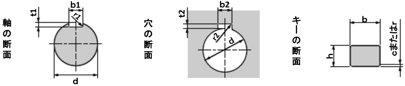
JIS (JIS B 1301-1976抜粋)
